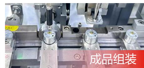
转子推送
